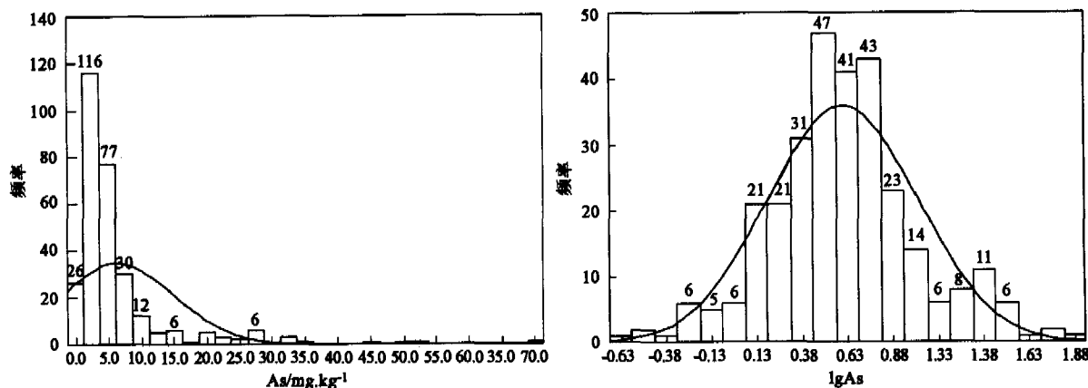
图 1 中国煤中砷含量分布图
