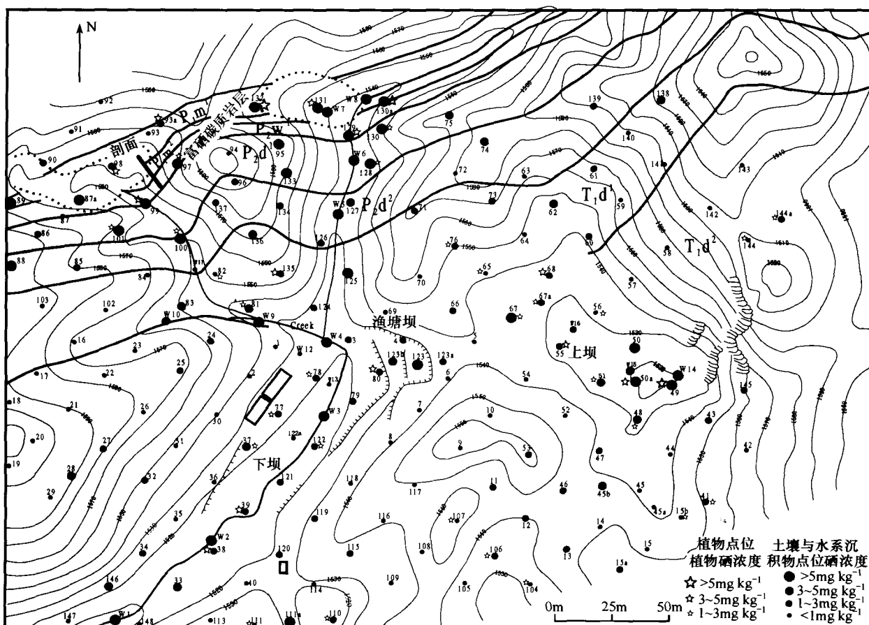
图 1 渔塘坝简明地质地形及采样点与点位土壤、植物硒含量分布图
