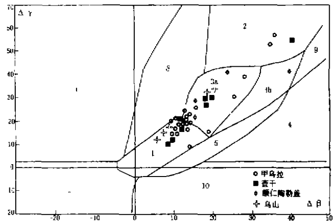
图 2 区域部分典型矿床矿石铅的 \Delta\beta - \Delta\gamma 成因分类图解 [1998, 朱炳泉] (部分原始数据据潘龙驹等, 1996)
