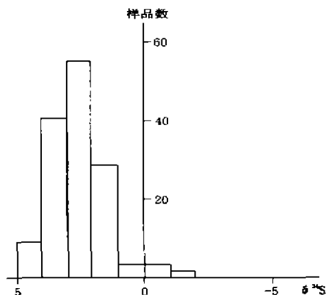
图 1 乌奴克吐山、甲乌拉、查干及额仁陶勒盖矿床 \delta^{34}\text{S} 频率直方图 (部分原始数据据潘龙驹等, 1996)
