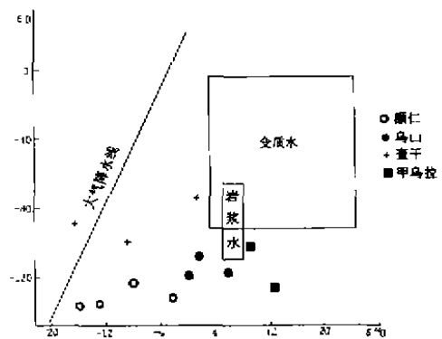
图 3 氢氧同位素成分图
