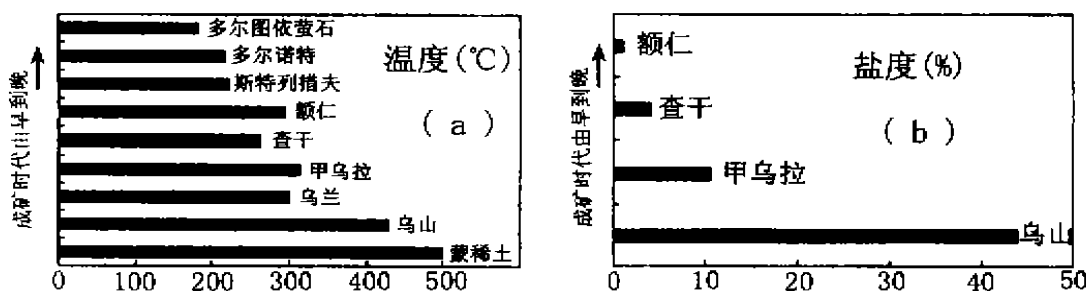
图 4 区域部分典型矿床石英包裹体均一化温度中值、盐度自早到晚变化图
