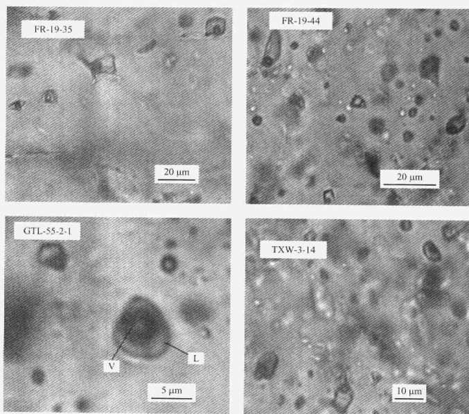
图 2 芙蓉锡矿田矿石流体包裹体
