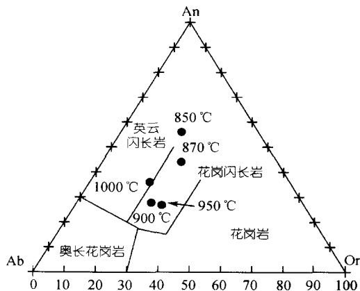
图 7 2.0 GPa, 恒温 12 h, 不同温度条件下的熔体 Ab~An~Or 图
