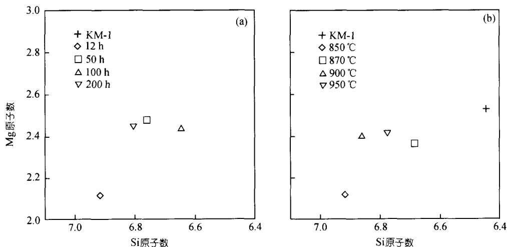
图2 角闪石的 Si-Mg 图
