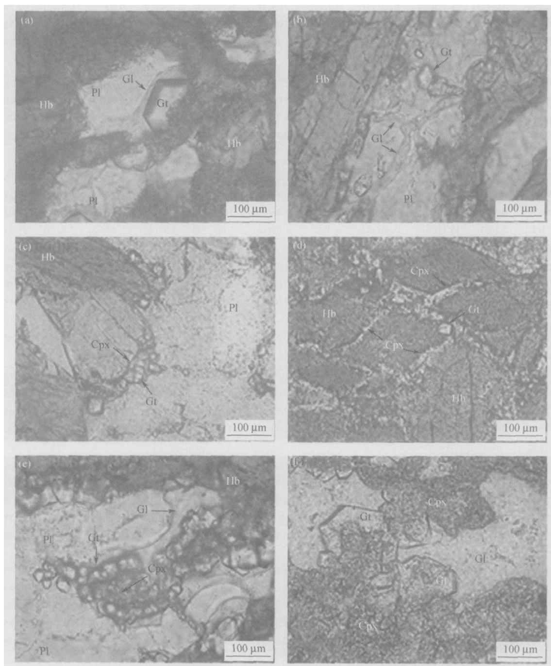
图 1 实验产物的显微照片
