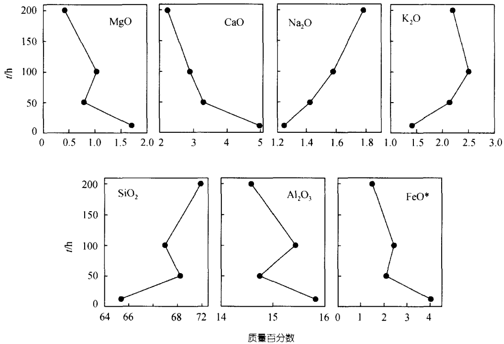
图 4 2.0 GPa, 850°C, 不同加热时间对熔体成分的影响
