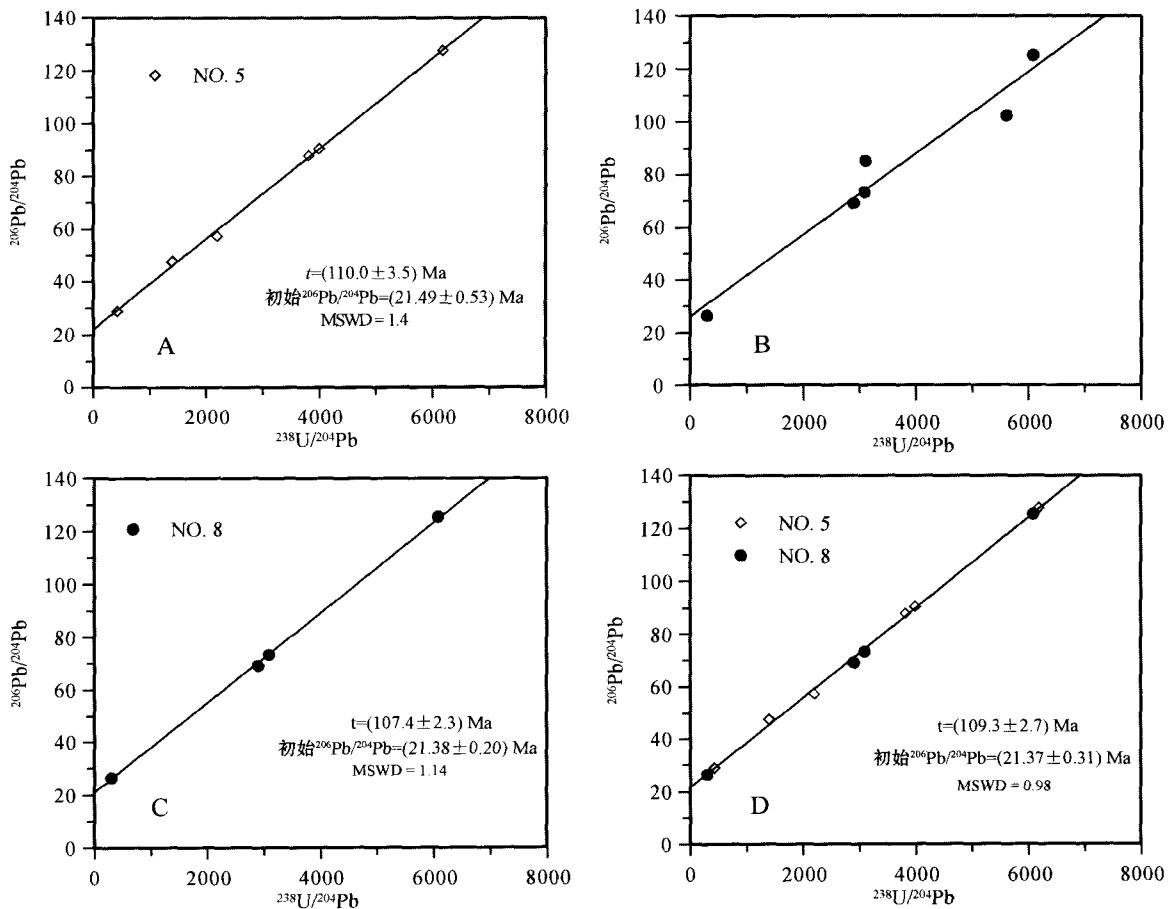
图 2 661 铀矿床矿石 U-Pb 等时线图
