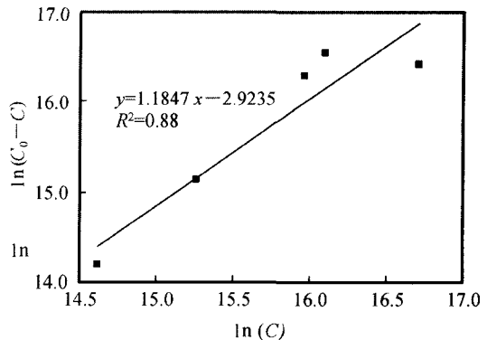
图 8 施氏矿物吸附 A. f 的 Freundlich 模型拟合 Fig. 8 Freundlich fitting of A. f adsorption on schwertmannite
