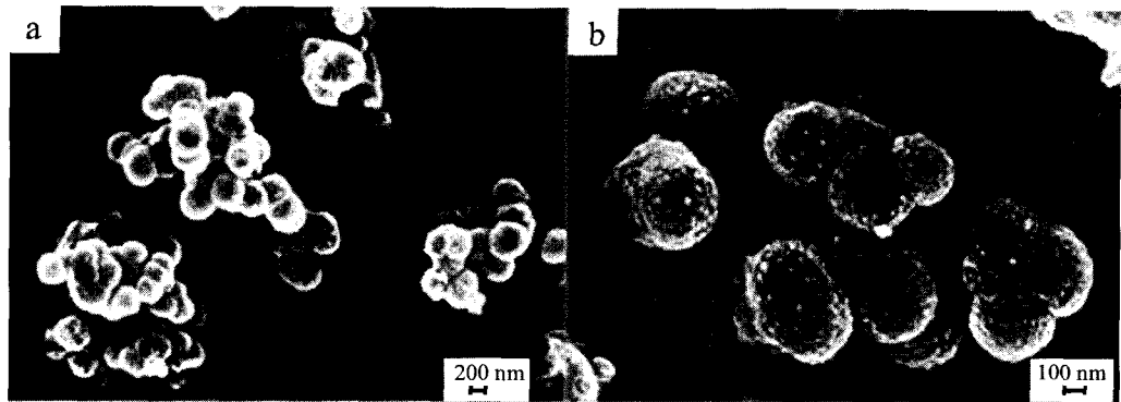
图2 施氏矿物的SEM照片 Fig. 2 SEM images of synthetic schwertmannite
