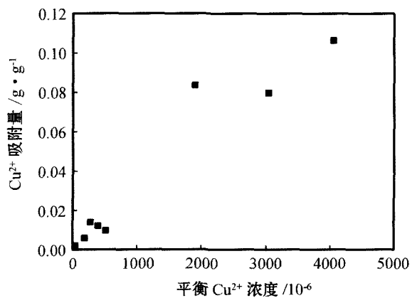
图4 施氏矿物对 Cu 2+ 的吸附等温线 Fig. 4 Adsorption isotherm of Cu 2+ on schwertmannite
