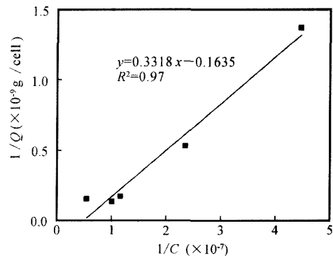
图 7 施氏矿物吸附 A. f 的 Langmuir 模型拟合 Fig. 7 Langmuir fitting of A. f adsorption on schwertmannite
