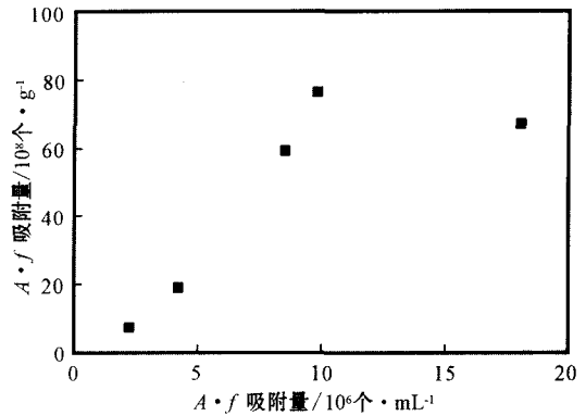
图 6 施氏矿物对 A. f 菌的吸附等温线 Fig. 6 Adsorption isotherm of A. f on schwertmannite
