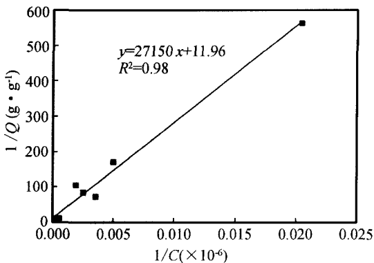
图 5 施氏矿物吸附 Cu^{2+} 的 Langmuir 模型拟合 Fig. 5 Langmuir fitting of Cu^{2+} adsorption on schwertmannite
