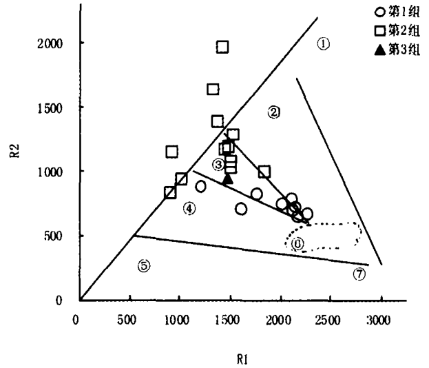
图 13 侵入岩形成构造环境的主量元素 R1 ~ R2 因子判别图(据 Batchelor 等,1985)
