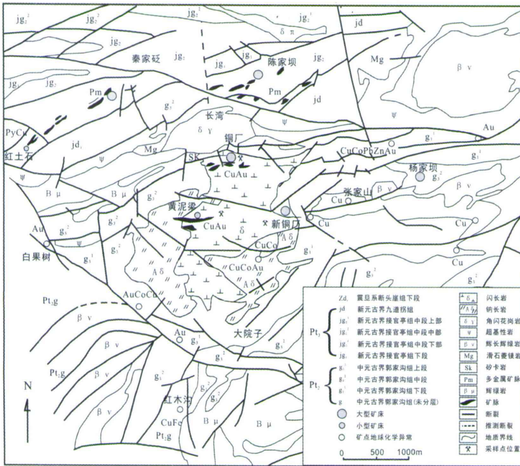
图1 铜厂矿田地质图(据西北有色地堪局711队1994图件和李军,1990修绘)
