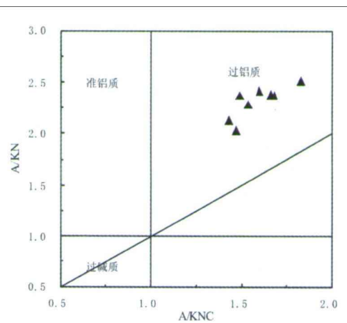
图2 铜厂闪长岩铝饱和指数(山德理指数)图解
