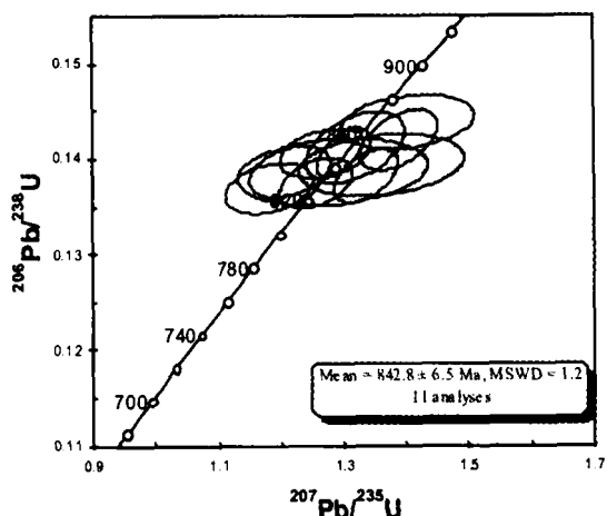
图8 铜厂闪长岩锆石 SHRIMP U-Pb 年龄谱和图
