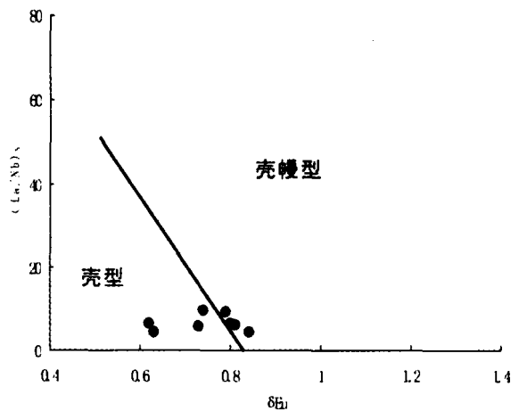
图 14 铜厂闪长岩的 (La/Yb)_N - \delta Eu 关系图(据邵拥军等, 2003)
