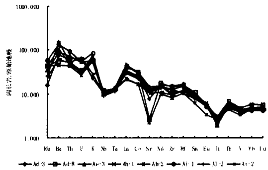
图 4 铜厂闪长岩不相容元素原始地幔标准化蛛网图
