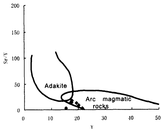
图9 铜厂闪长岩 Y-Sr/Y 图 (据 Defant&Drummond, 1993; Defant et al. , 2002)
