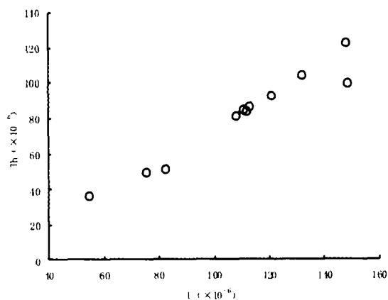
图7 铜厂闪长岩锆石 Th-U 图解
