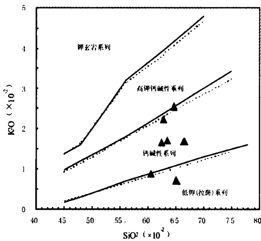
图 3 铜厂闪长岩 K_2O-SiO_2 图解
