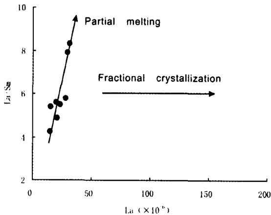
图 15 铜厂闪长岩的 La-La/Sm 图解 (据 Allegre et al. , 1978; Lai et al. , 2003)
