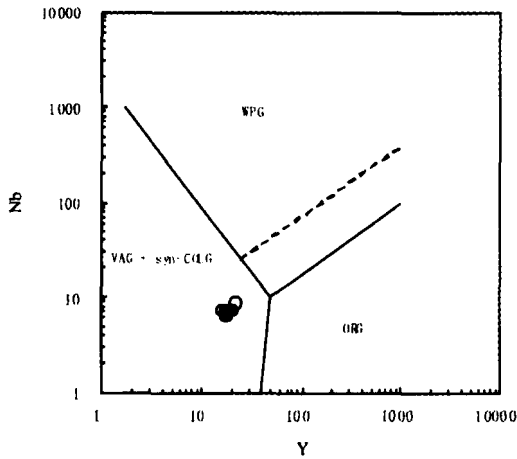
图 11 铜厂闪长岩 Nb-Y 图(据 Pearce 等,1984)
