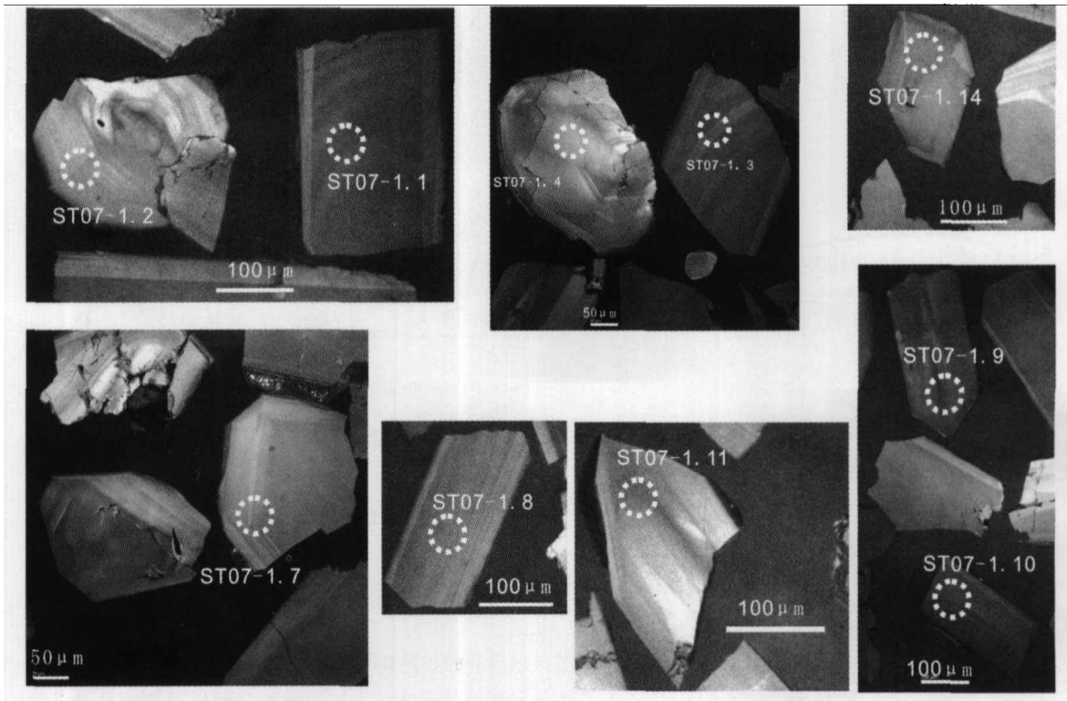
图 6 铜厂闪长岩锆石 CL 图像和测点位置
