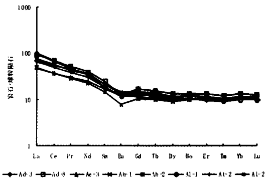
图 5 铜厂闪长岩稀土元素球粒陨石标准化配分图
