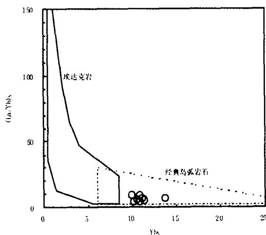
图10 铜厂闪长岩 Yb_N-(La/Yb)_N 图 (据 Drummond et al. , 1990)
