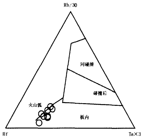
图 12 铜厂闪长岩 Rb/30-Hf-Ta x 3 图解
