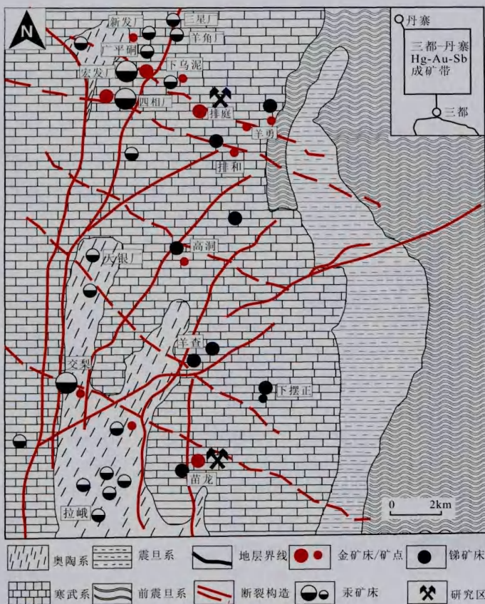
图 1 贵州三都-丹寨汞-金-锑矿化带地质构造简图(据高振敏等,2002 修改)
