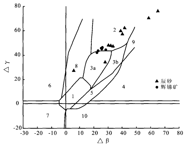
辰砂和部分辉锑矿数据据何立贤等(1993);1-地幔源铅;2-上地壳源铅;3-上地壳与地幔混合的俯冲带铅;3a-岩浆作用;3b-沉积作用;4-化学沉积型铅;5-海底热水作用铅;6-中深变质作用铅;7-深变质作用下地壳铅;8-造山带铅;9-古老页岩上地壳铅;10-退变质作用铅
