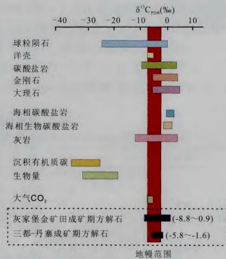
灰家堡金矿田数据据王泽鹏等(2012)及部分未发表数据
