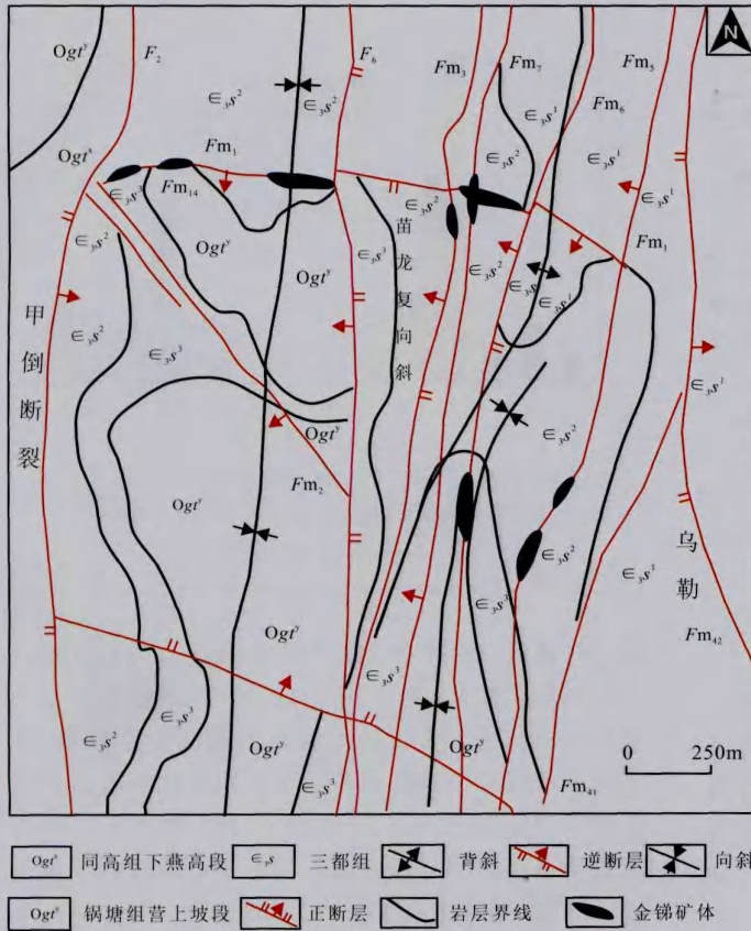
图3 苗龙金锑矿床地质构造简图(据王尚彦等,2006)
