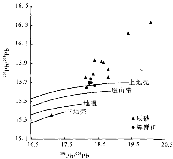
辰砂和部分辉锑矿数据据何立贤等(1993) 图 8 三都—丹寨成矿带辰砂、辉锑矿铅同位素组成(底图据 Zartman and Doe, 1981 修改)
