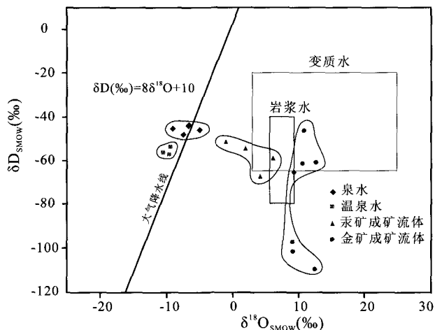
原始数据据陈庆年等,1998;高振敏等,2002;严钧平等,1989, \delta^{18}\text{O}_{\text{H}_2\text{O-SWOM}} 是采用同位素平衡分馏方程计算而得出来的, \delta^{18}\text{O}_{\text{H}_2\text{O-SWOM}} = \delta^{18}\text{O}_{\text{SWOM}} - A * 10^6 T^{-2} - B 。其中当测定矿物为石英时: A=3.38, B=-3.4 ;方解石: A=2.78, B=-3.4 ;白云石: A=3.20, B=-3.4
