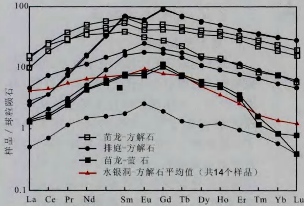
图4 与成矿有关的方解石、萤石稀土元素标准化配分模式图(水银洞数据据夏勇等,2009)
