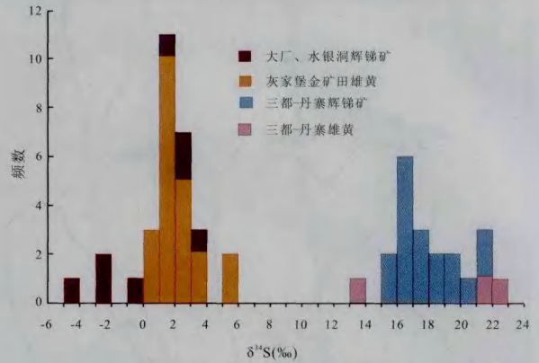
三都-丹寨雄黄和部分辉锑矿数据据陈庆年等(1998); 黔西南数据据张瑜等(2010)及部分未发表数据
