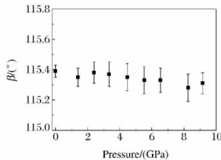
图 4 绿帘石 \beta 值随压力的变化
