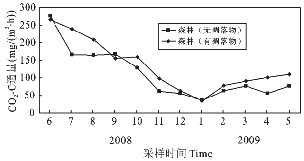
图 3 森林土壤在有或无凋落物条件下的 CO 2 -C 通量季节变化
