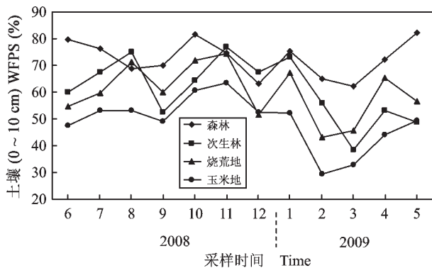
图 6 不同土地覆被下土壤 WFPS(0~10 cm)的季节变化
