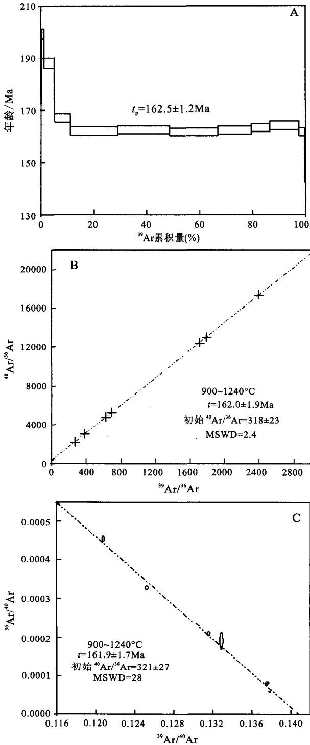
图3 样品 SYBLTS-01 白云母坪年龄(A)、等时线年龄(B)、反等时线年龄(C)
