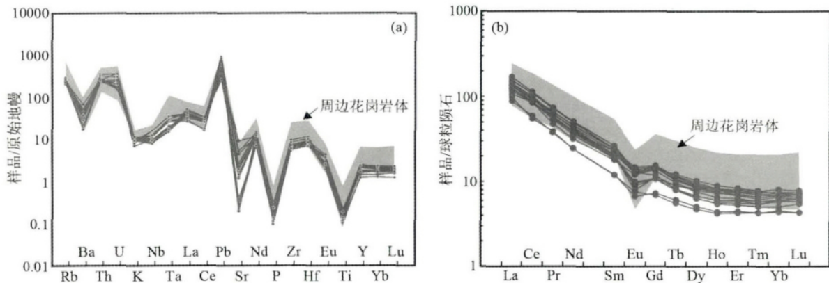
图4 脉岩的原始地幔标准化微量元素蛛网图(a, 标准化值据 Sun and McDonough, 1989) 和球粒陨石标准化稀土元素分布型式图(b, 标准化值据 Taylor and McLennan, 1985)
