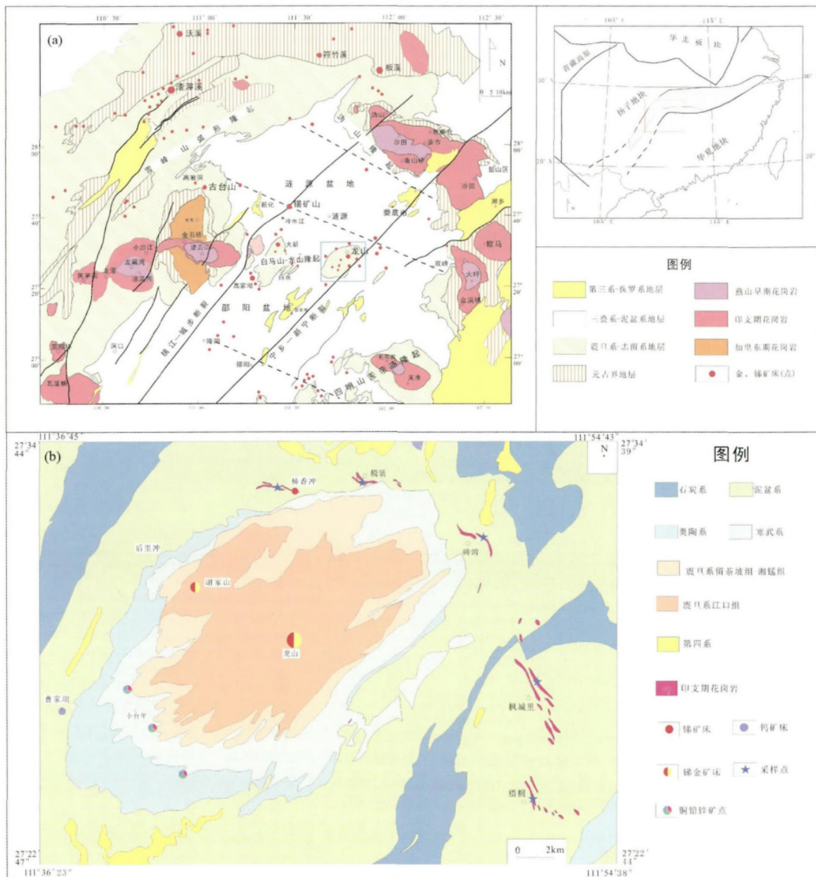
图 1 湘中地区地质图 ( a,据陶琰等, 2001; 李己华等, 2007 修改) 和龙山金锑矿区地质图 ( b,据贺文华等, 2015)
