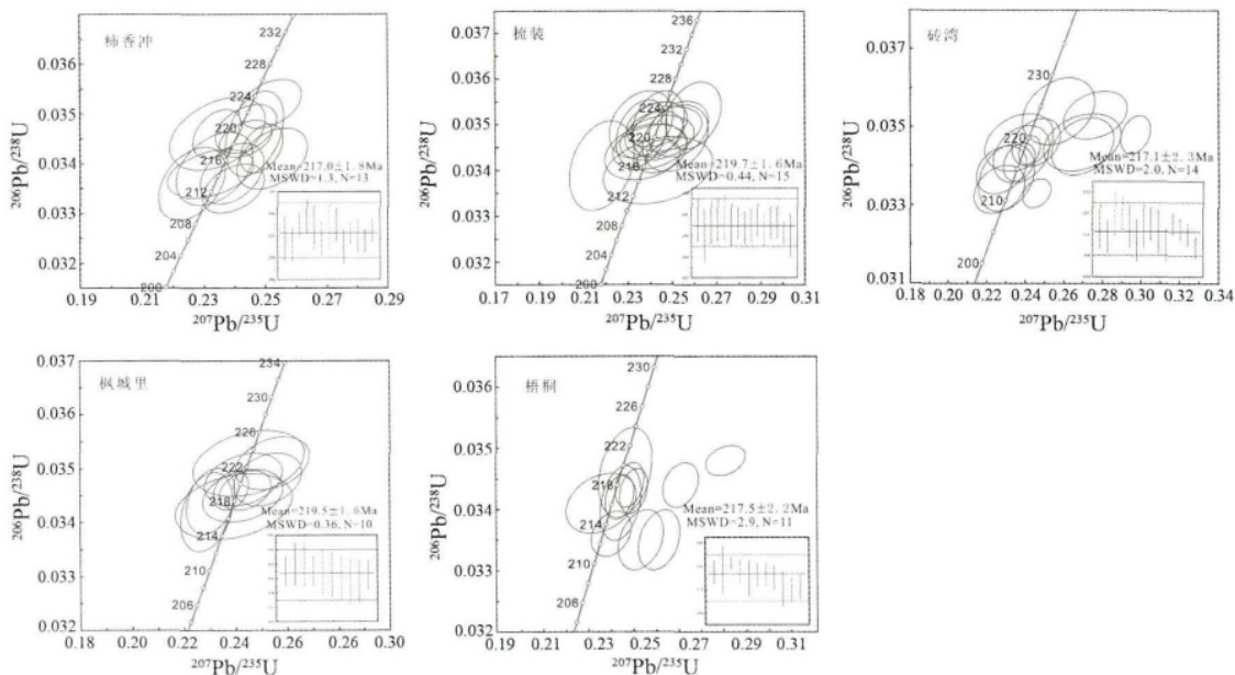
图 3 岩脉的锆石 U-Pb 谐和图
