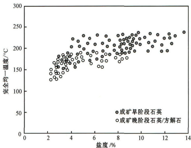
图8 包裹体均一温度对盐度图解
