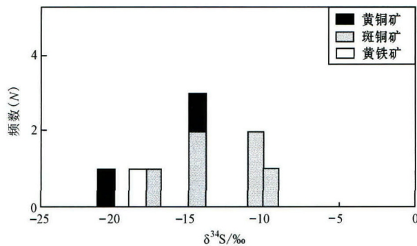
图 7 科登涧铜矿床 S 同位素组成图解
