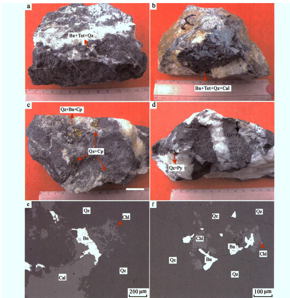
图3 科登涧铜矿床矿物组合手标本及镜下照片
