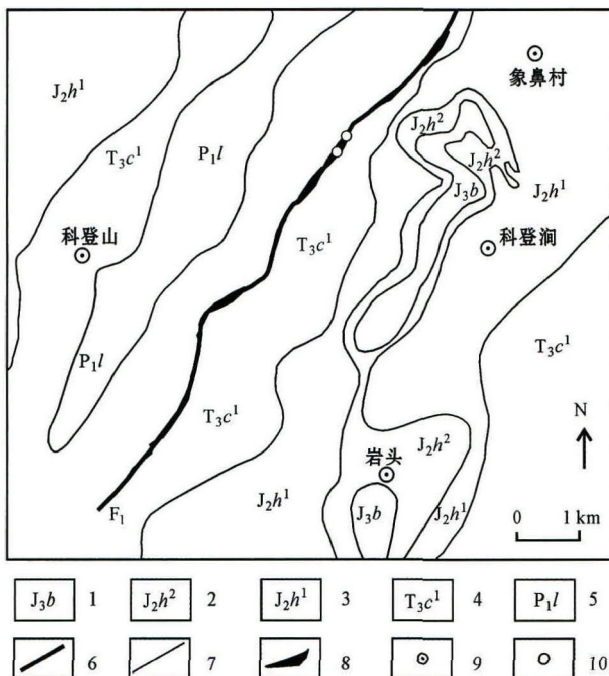
图2 科登涧铜矿床地质简图(据李永森,2002)
