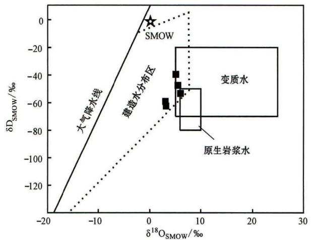
图 6 科登涧铜矿床 H、O 同位素组成图解 (底图据郑永飞等 2000)
