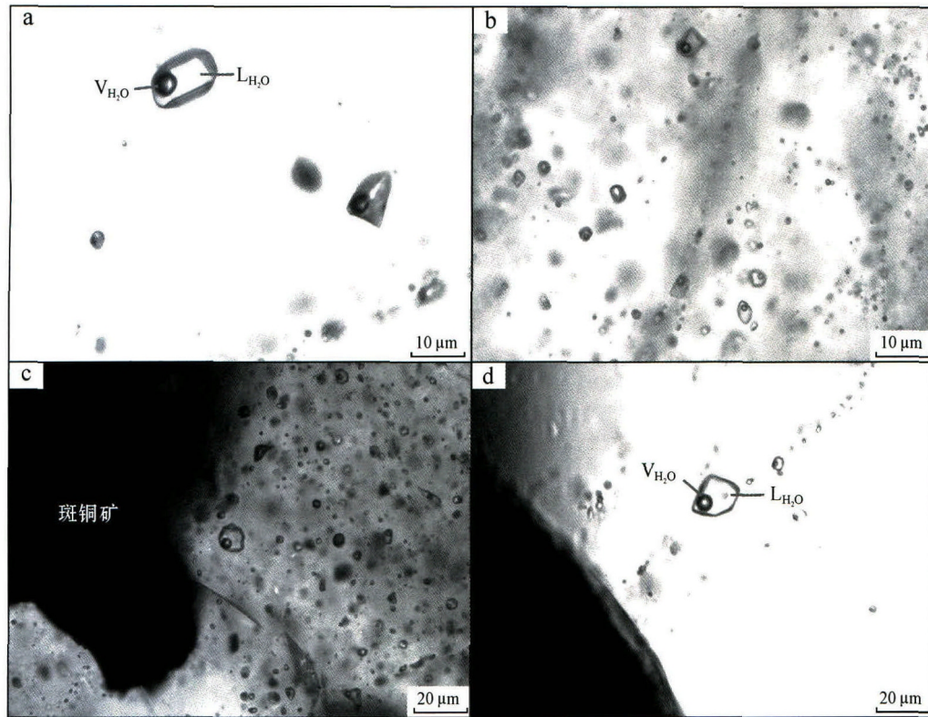
图4 科登涧铜矿床包裹体照片
