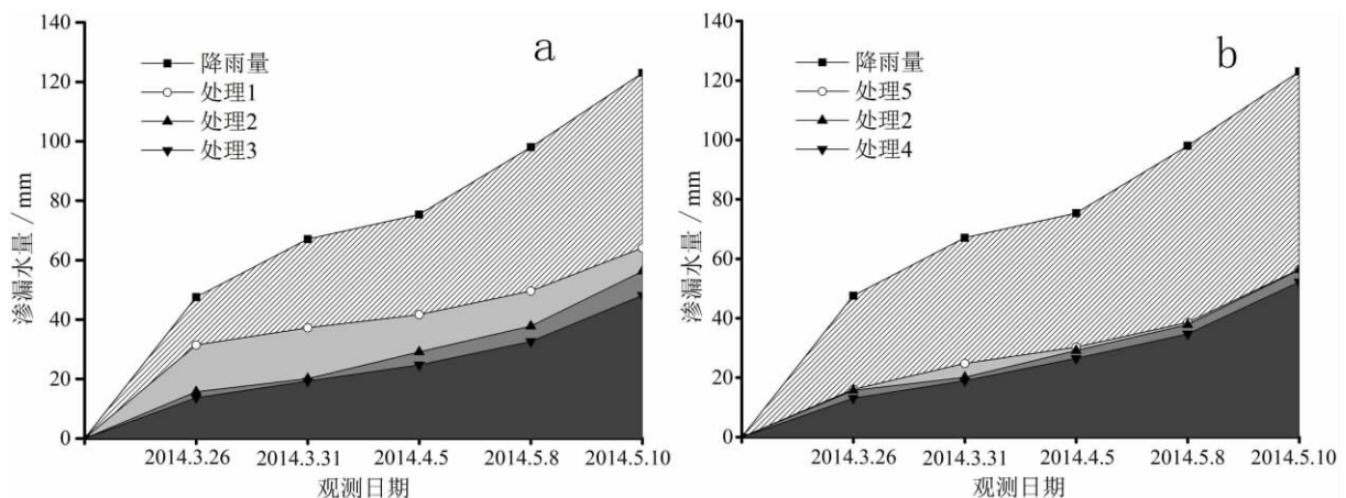
图 1 保水剂(a)和活性炭(b)对土壤渗漏水量的影响
