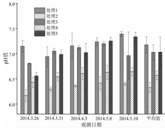
图 2 保水剂和活性炭对土壤渗漏水 pH 值的影响
