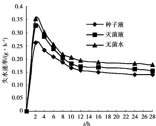
图 3 45 °C 下土壤的失水速率
