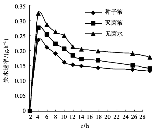
图 2 28 °C 下土壤的失水速率
