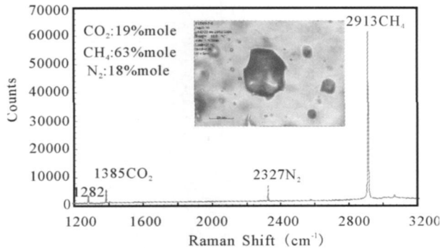
图 9 气相 CH 4 -N 2 -CO 2 (L CH 4 +N 2 +CO 2 ) 包裹体及激光拉曼光谱
