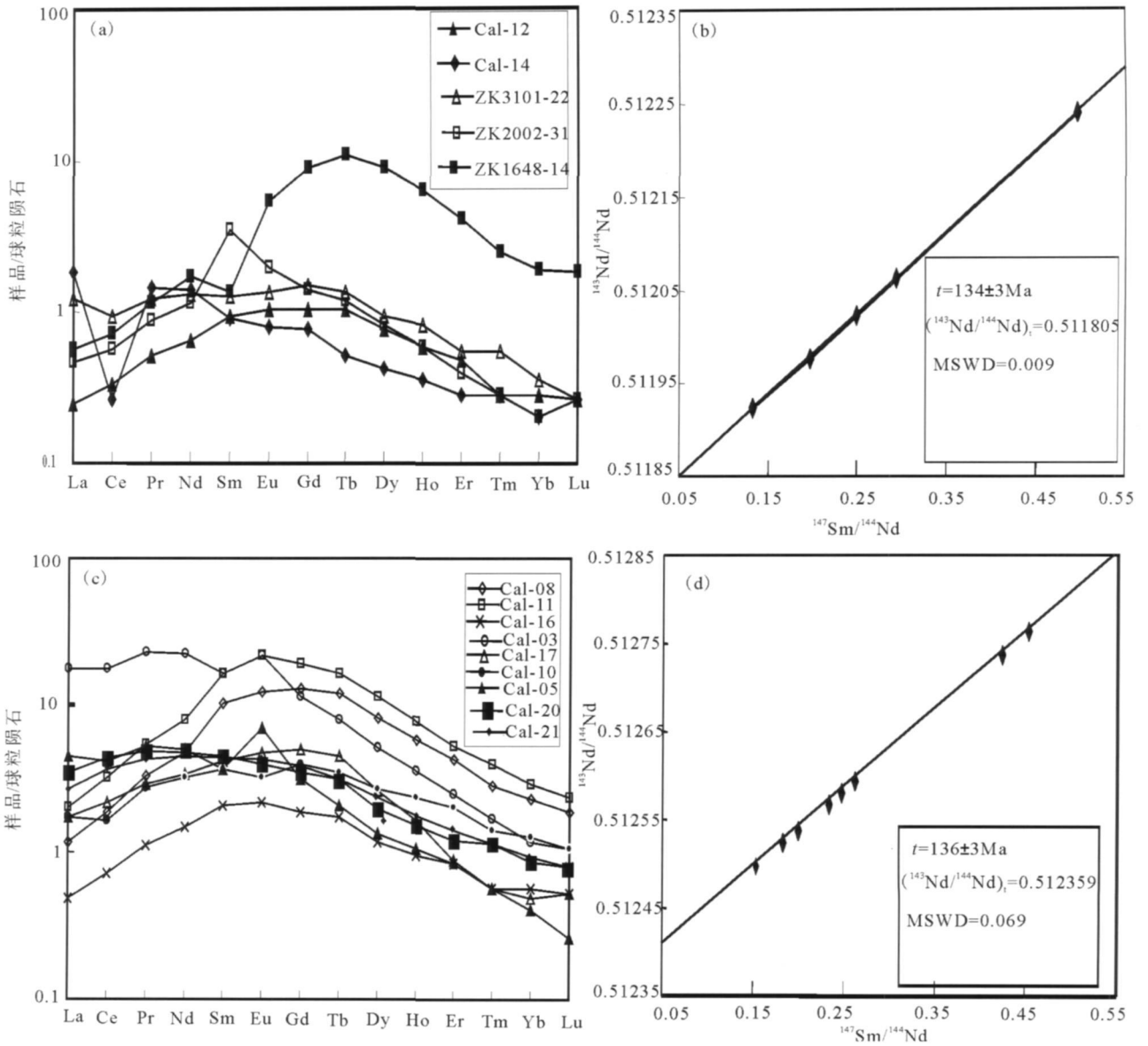
图 6 黔西南水银洞金矿方解石脉 REE 模型(a,c)和对应的 Sm-Nd 同位素年龄(b,d)(据 Su 等, 2009)
