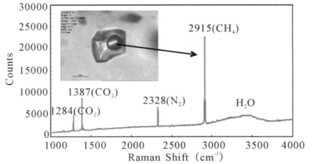
图 10 气液相 V CH 4 +N 2 +CO 2 +H 2 O 包裹体及激光拉曼光谱 Fig. 10 Gas-liquid V CH 4 +N 2 +CO 2 +H 2 O inclusion and the laser Raman spectra
