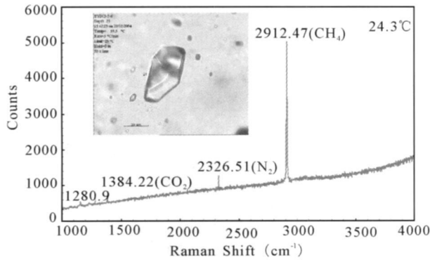
图 8 液态 CH 4 -N 2 -CO 2 (L CH 4 +N 2 +CO 2 ) 包裹体及激光拉曼光谱
