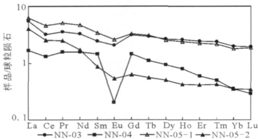
图 5 黔西南水银洞金矿床区域上与金矿无关的方解石脉稀土元素球粒陨石标准化型式
