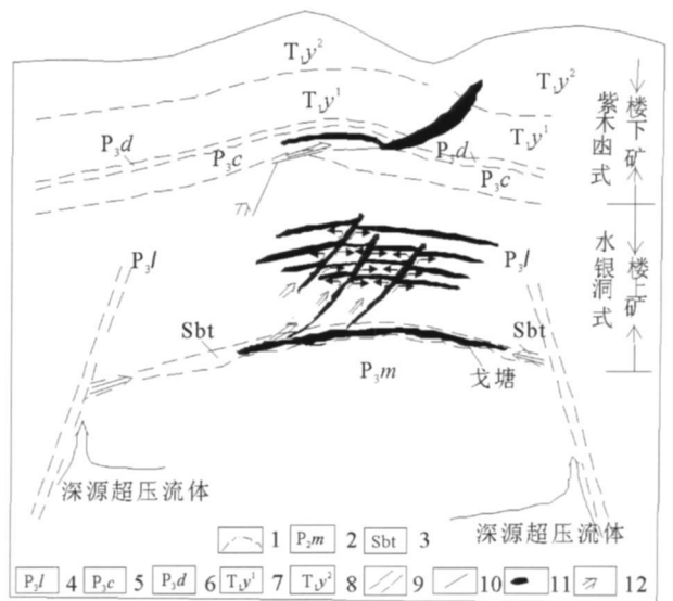
图 11 黔西南水银洞层控卡林型金矿床“两层楼”矿体分布及成矿模式示意图
