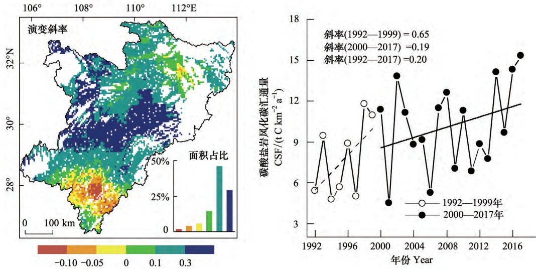
图 7 1992—2017 年槽谷年均碳酸盐岩风化碳汇通量演变空间分布及整体演变趋势
