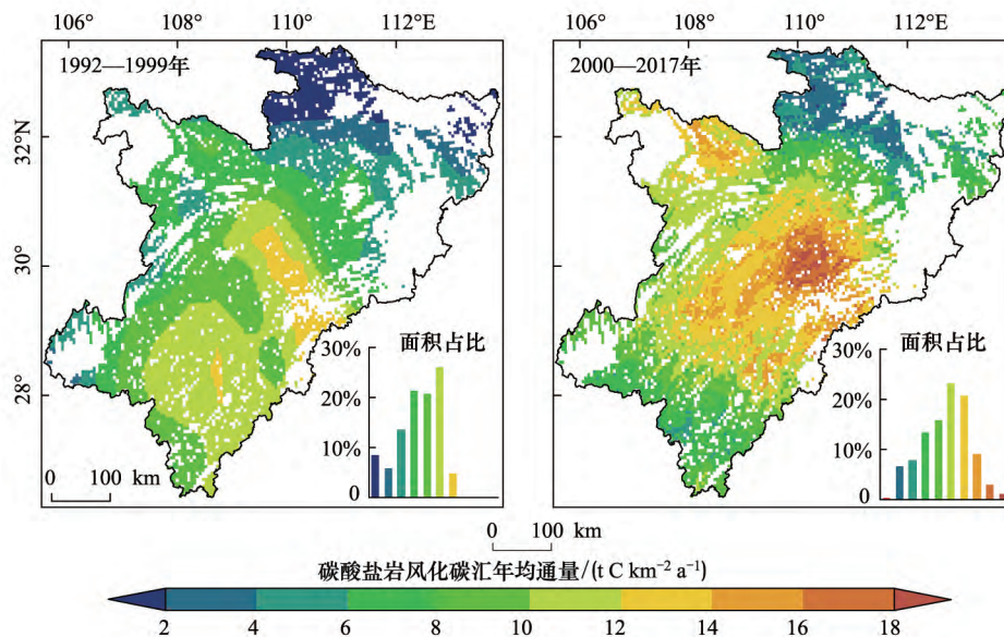
图6 1992—1999及2000—2017年槽谷碳酸盐岩化学风化碳汇空间分布格局
