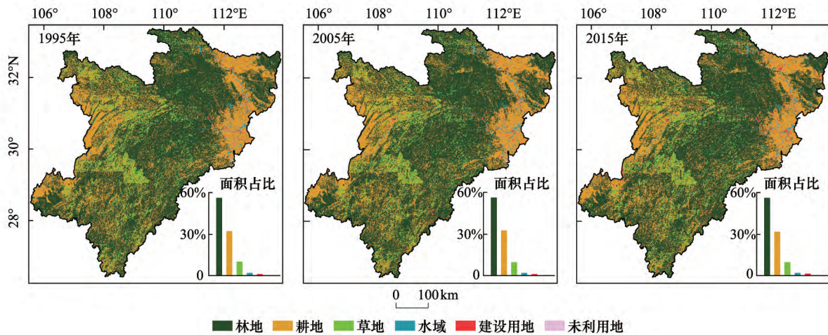
图5 槽谷1995年、2005年及2015年土地利用类型分布 Fig.5 Land cover/land use distributions of the valley in 1995, 2005 and 2015
