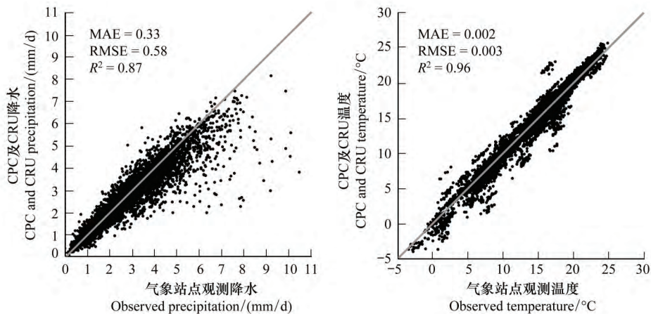
图10 美国国家海洋和大气管理局气候预报中心(CPC)及东英吉利大学气候研究中心(CRU)降雨及温度产品数据与中国气象局地面观测数据的对比,其中MAE为平均绝对偏差,RMSE为均方根误差
