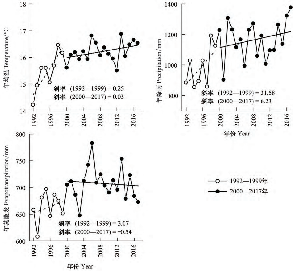
图2 喀斯特槽谷气候水文时间演变特征
