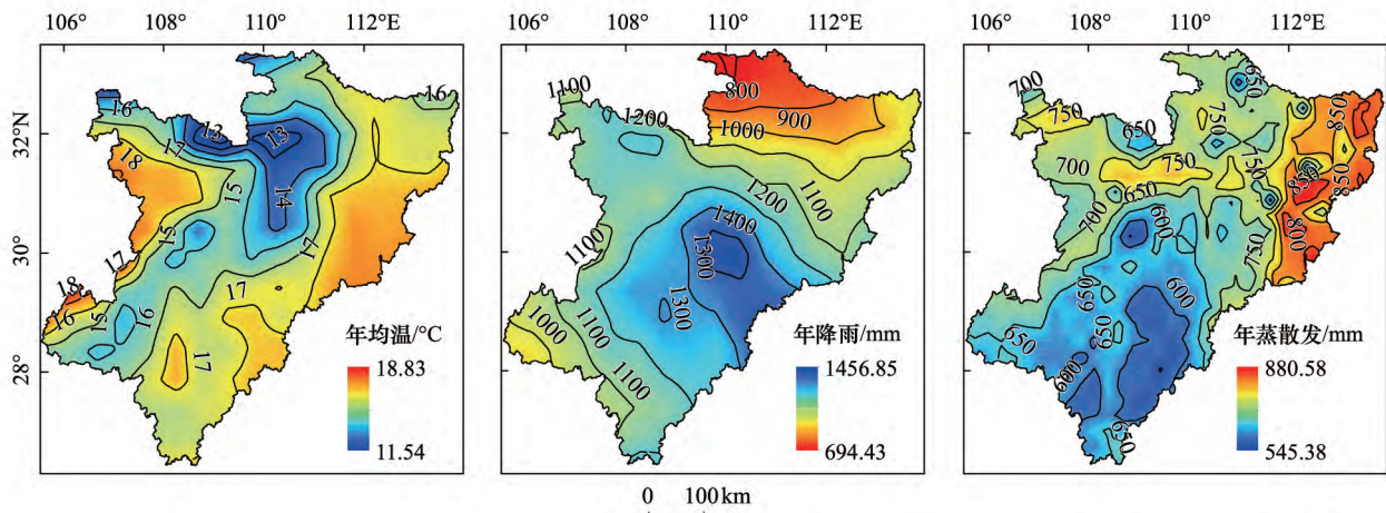
图 1 喀斯特槽谷气候水文空间分布特征
