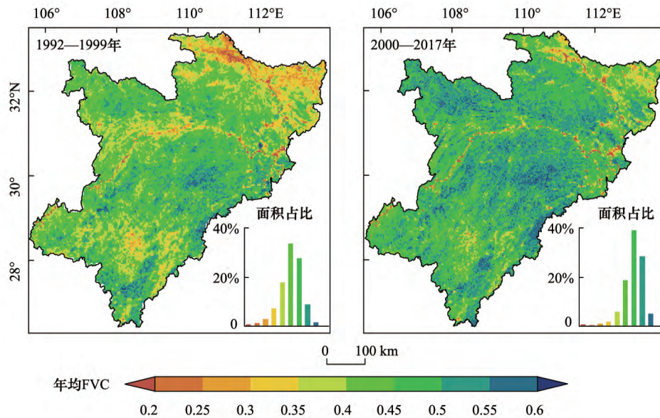
图3 槽谷 1992—1999 年及 2000—2017 年年均植被覆盖度(FVC)空间分布
