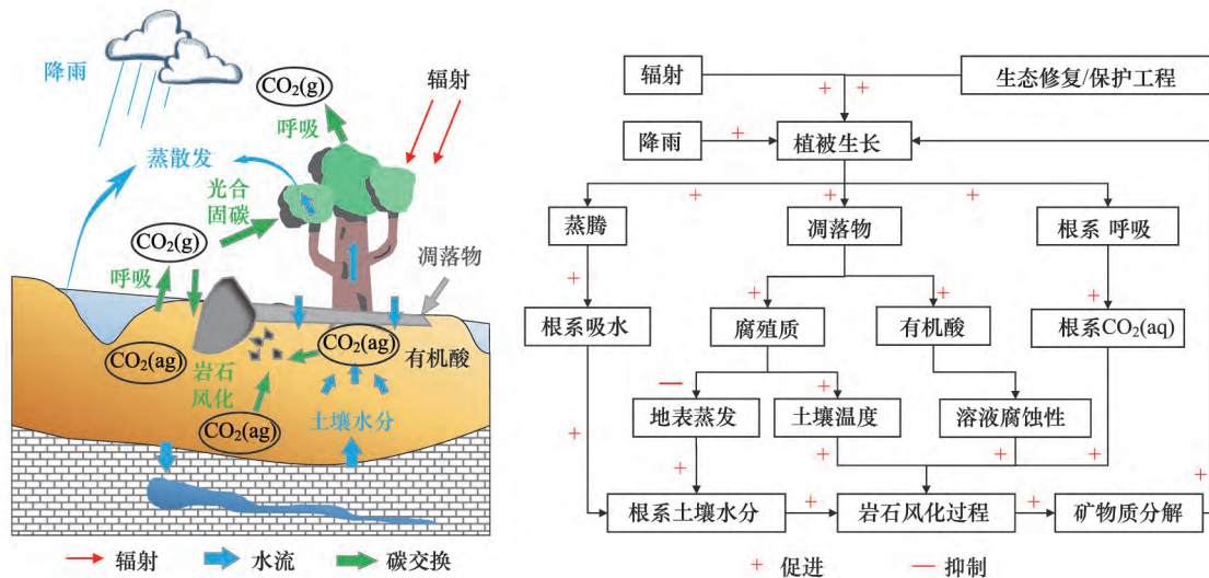
图9 气候变化及植被恢复对岩石风化过程的复合影响机制
