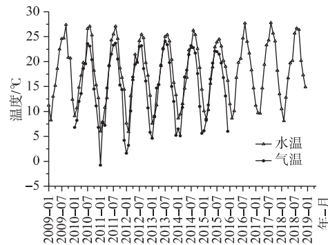
图 4 2009—2018 年红枫湖水温和气温变化趋势
