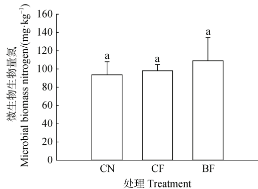
图 2 不同施肥处理下土壤微生物生物量氮 Fig. 2 Soil microbial biomass nitrogen in different treatments
