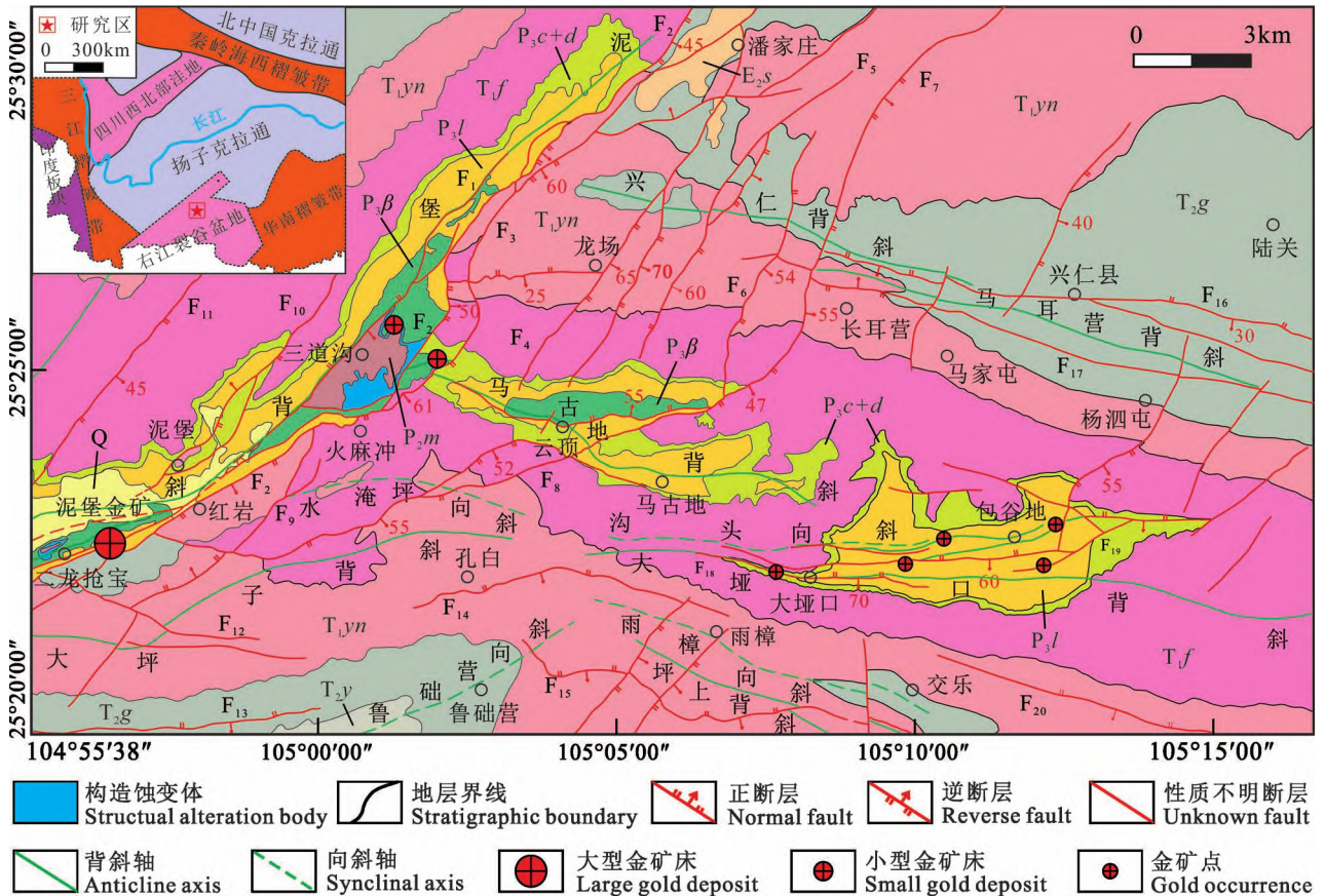
图 1 泥堡—包谷地卡林型金矿田地质矿产图(据李松涛等, 2021)
