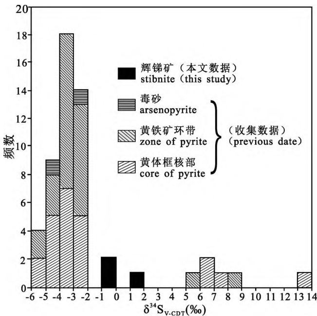
图 10 黔西南卡林型金矿辉锑矿、毒砂、环带状黄铁矿硫同位素频数图(数据来自本文; Wei Dongtian et al., 2020; 郑禄林等, 2019)
