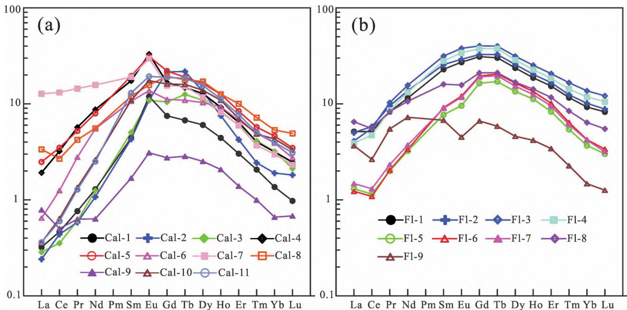
图 5 黔西南泥堡—包谷地卡林型金矿田方解石(a)、萤石(b)中稀土元素球粒隕石标准化分布型式图
