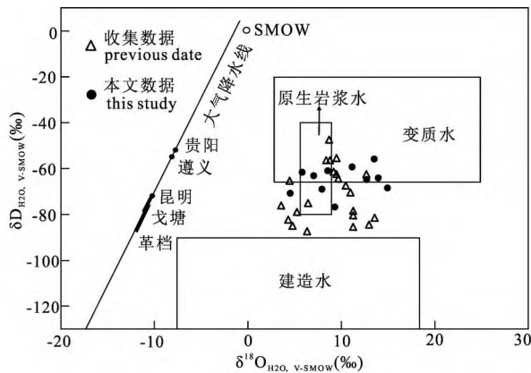
图 8 黔西南卡林型金矿石英—流体氢氧同位素 \delta^{18}\text{O}_{\text{H}_2\text{O}, \text{V-SMOW}} - \delta\text{D}_{\text{H}_2\text{O}, \text{V-SMOW}} 图解 (底图据 Hu Ruizhong et al., 2017, 数据来自本文; Li Songtao et al. 2019; 谢贤洋等, 2016; 吴松洋等, 2016; 郑禄林等, 2019)
