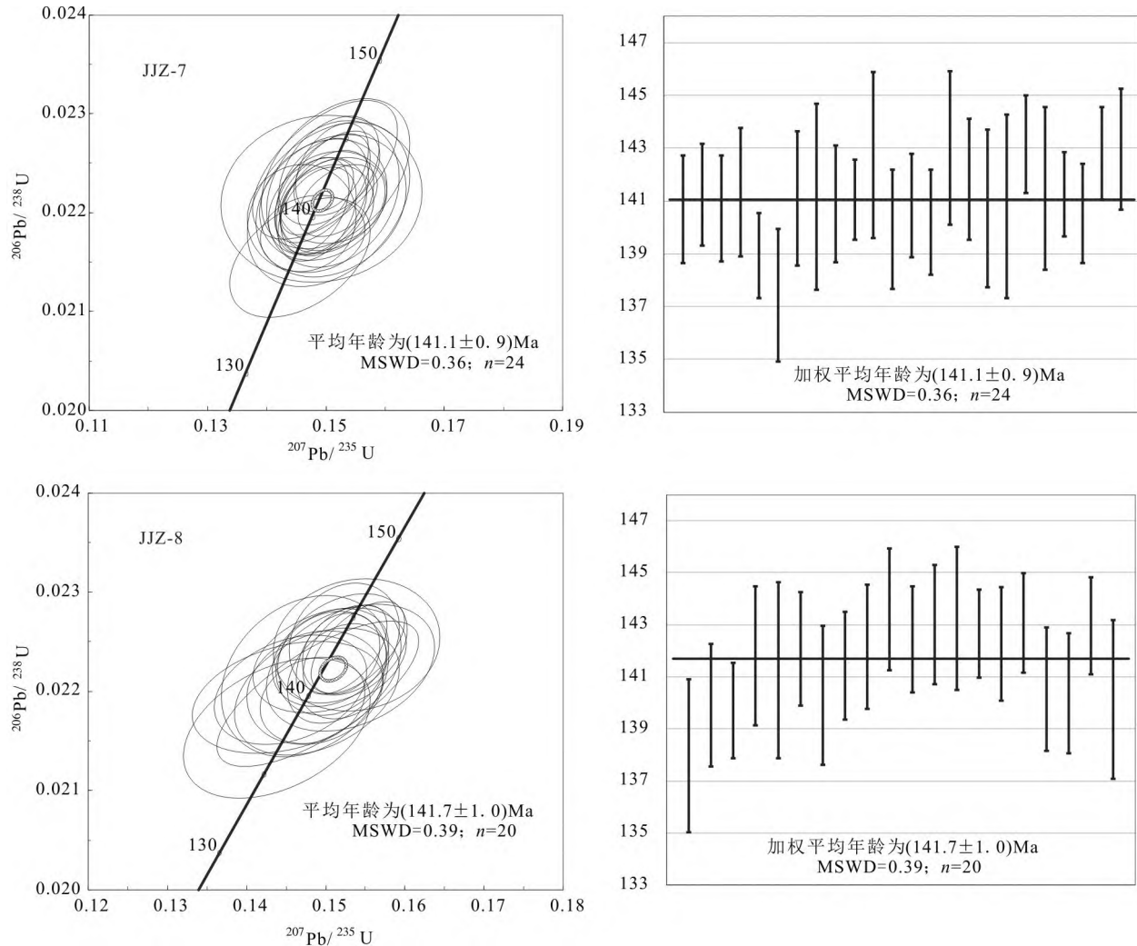
图7 金井咀金矿闪长岩锆石U-Pb年龄谱和图
