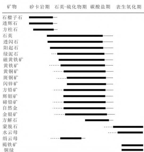
图5 金井咀矿床矿物生成序列图
