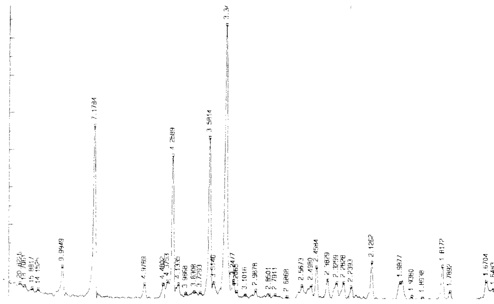
图5 高岭石加绢云母型粘土 XRD 谱图
