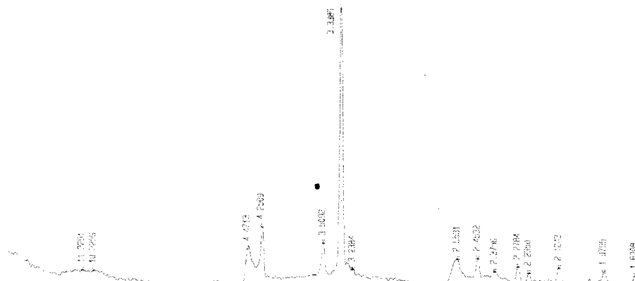
图4 石英型粘土 XRD 谱图
