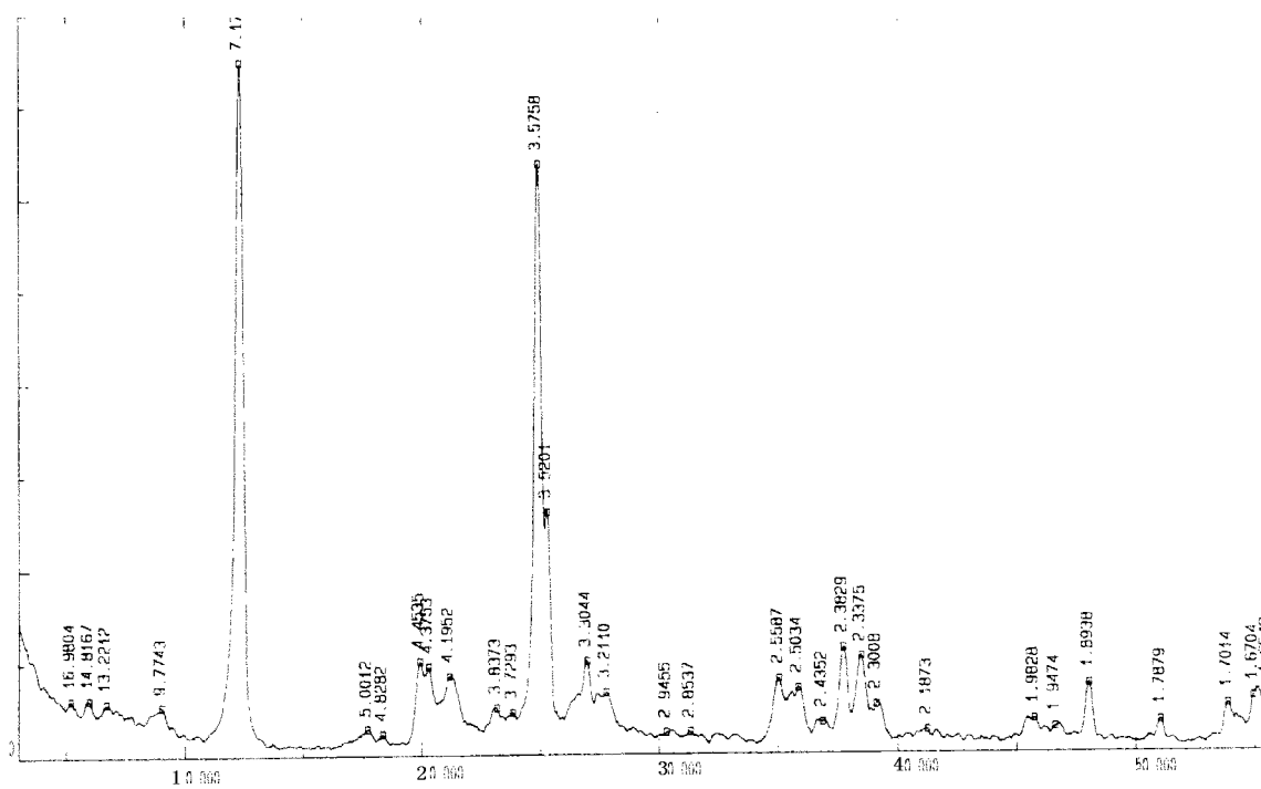
图 1 高岭石型粘土 XRD 谱图
