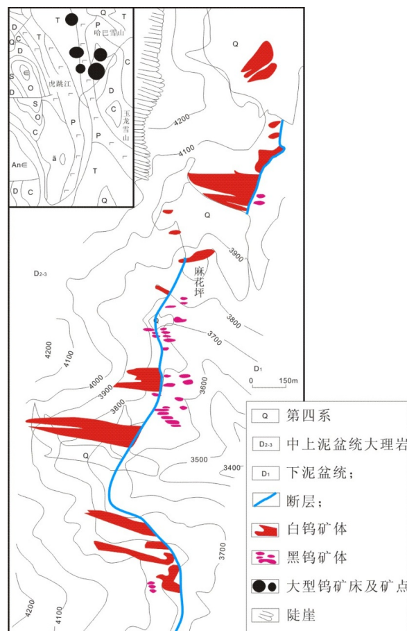
图 1 中甸县麻花坪钨铍矿矿体分布图(据冉明佳等, 2011)
