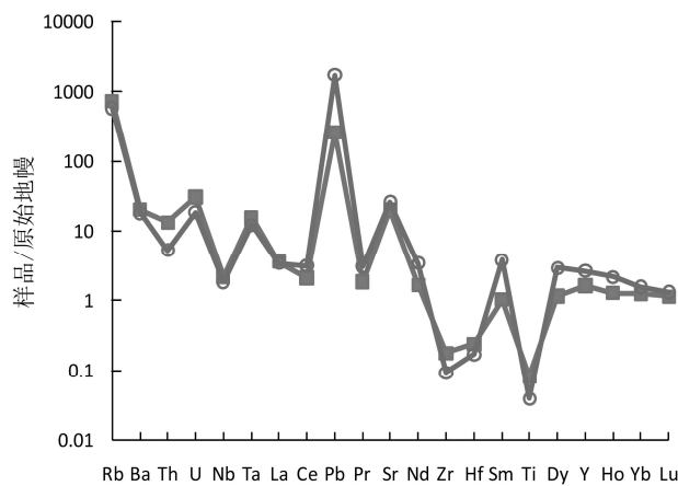
图 2 麻花坪钨铍矿矿石微量元素蛛网图
