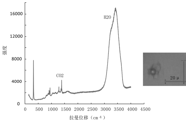
图 3 麻花坪伟晶岩萤石中流体包裹体激光拉曼光谱
