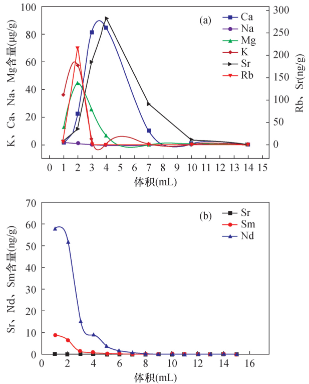
图 3 (a) AG50W - X8 树脂以 2 mol/L 硝酸洗脱 Sr 的曲线; (b) AG50W - X8 树脂以 6 mol/L 硝酸洗脱 REEs 的曲线
