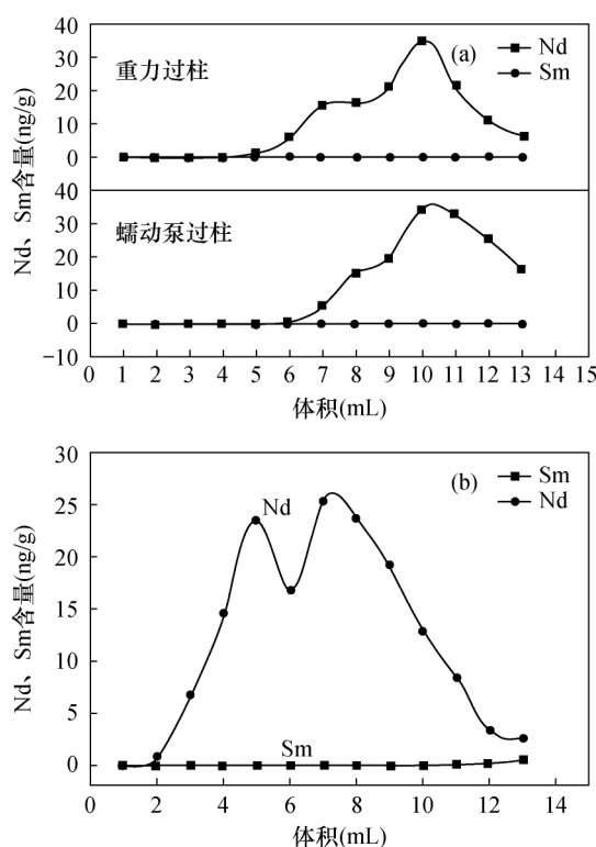
图5 (a) Ln特效树脂采用不同过柱方式对Sm和Nd的洗脱曲线;(b) Ln特效树脂最佳条件下洗脱Nd元素曲线
