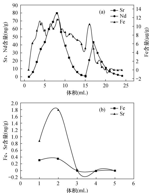
图 1 AG50W - X8 树脂 (a) 和 AG1 - X8 树脂 (b) 对 Fe 的淋出曲线
