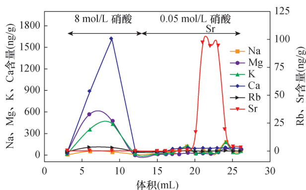
图4 Sr特效树脂洗脱Sr曲线
