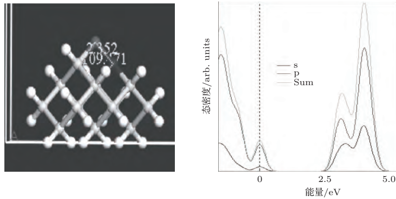
图 5 在硅量子点的弯曲表面上键合的 Si—NO 键结构及其态密度分布
