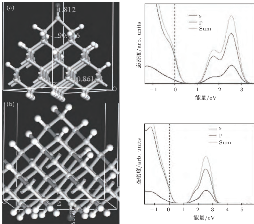
图 6 (a) 在同样大小的硅量子点的弯曲表面上键合的 Si=O 双键结构及其态密度分布; (b) 在同样大小的硅量子点的小平台表面上键合的 Si=O 双键结构及其态密度分布
