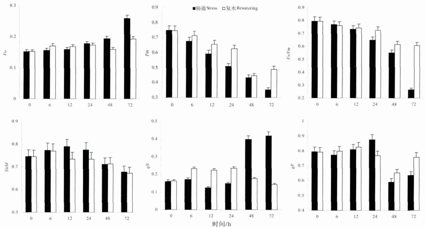
图 1 模拟干旱和复水对反叶扭口藓叶绿素荧光参数的影响
